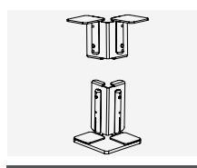
FF-90C Kit connettore a 90°
