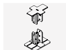
FF-CC Kit connettore a croce
