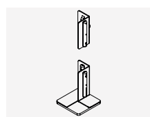
FF-90LIC Kit connettore interno sinistro a 90°
